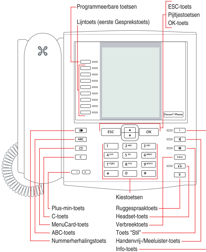
Toetsentoe wijzing aan de Forum Phone 536
